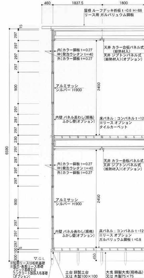
2階建標準断面図
