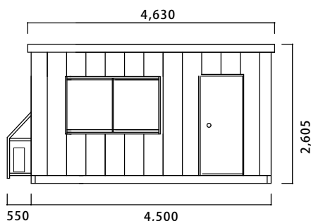
立面図 Elevation
