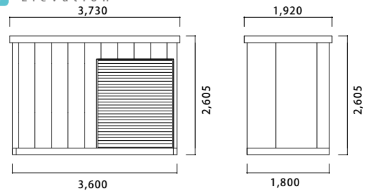
立面図 Elevation
