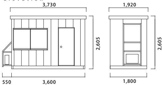
立面図 Elevation
