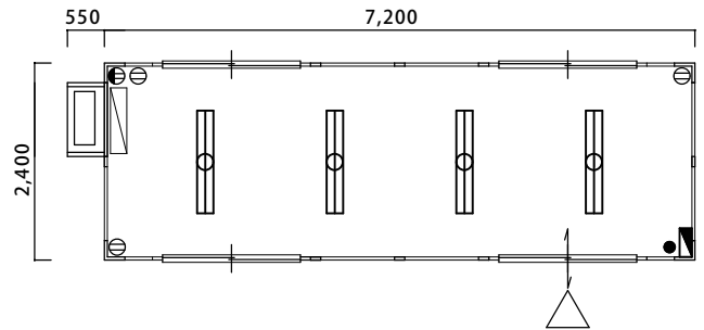
平面図
