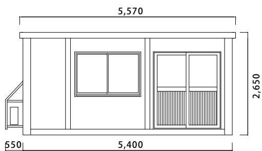
立面図 Elevation
