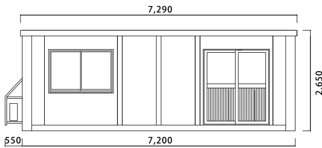
立面図
