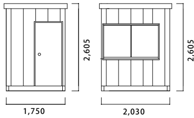
立面図 Elevation
