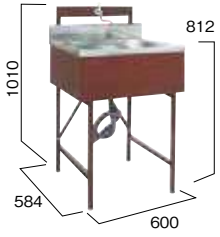
■1槽式 (重量16kg)
