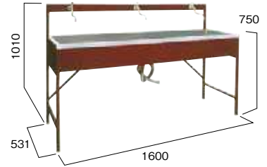
■全槽式 (重量24kg)
