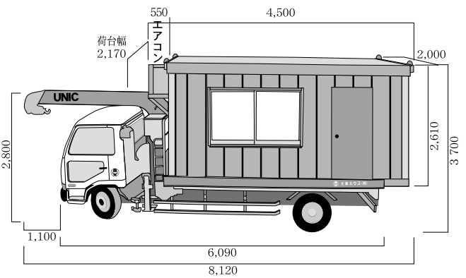
28型 * エアコン外機下部に取付タイプは、4t車による搬入・搬出となります。
