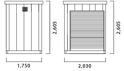
立面図 Elevation
